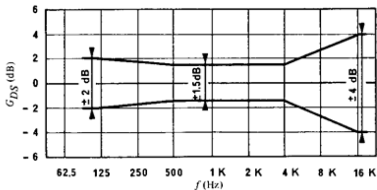
Сл. 1 - Дозволени толеранции за амплитудно-фреквенциската карактеристика на студиските мониторинг слушалки (според ITU препораката – ITU-R BS. 708)
