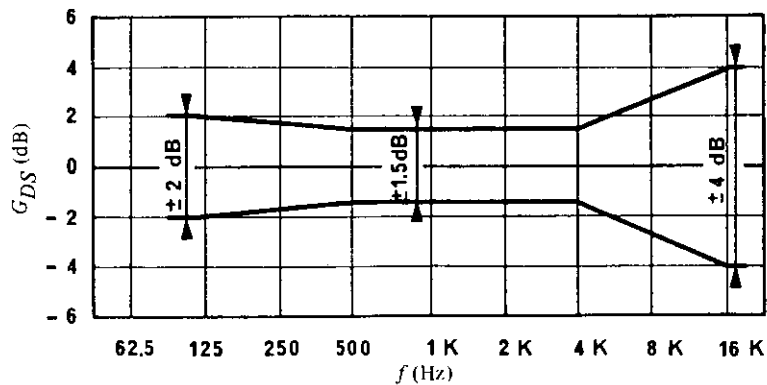
Сл. 1 - Дозволени толеранции за амплитудно-фреквенциската карактеристика на студиските мониторски слушалки (според ITU препораката – ITU-R BS. 708)
